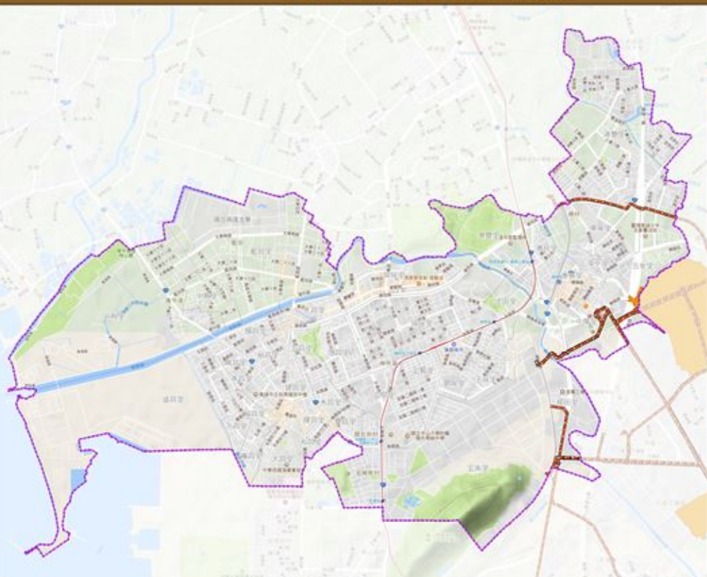
高雄市楠梓區工業管線分布圖
